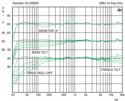
8260Aのフリーフィールド・レスポンスへのBASS TILT、TREBLE TILT、DESKTOP LOW FREQUENCY、BASS ROLL-OFFの各コントロールの効果
