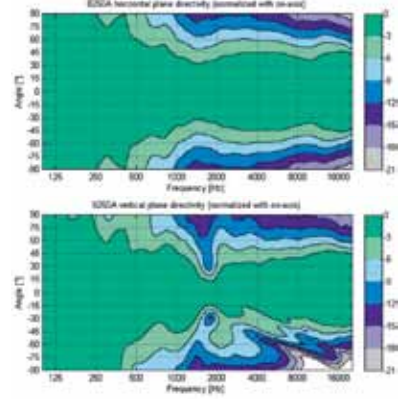
8250Aの水平指向性プロット (上)、垂直指向性プロット (下)
