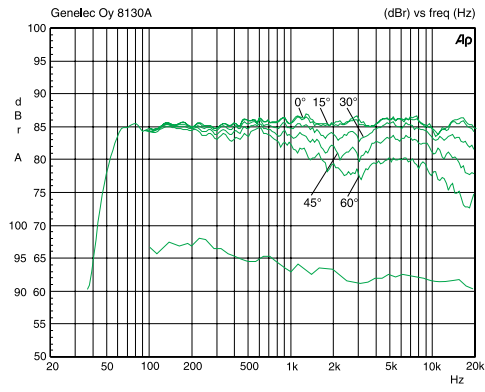
上側:8130Aの水平指向性特性(1m位置で計測)。下側:同システムのパワー・レスポンス
