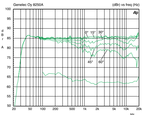
上側: 8250Aの水平指向性特性 (1 m 位置で計測)。下側: 同システムのパワー・レスポンス
