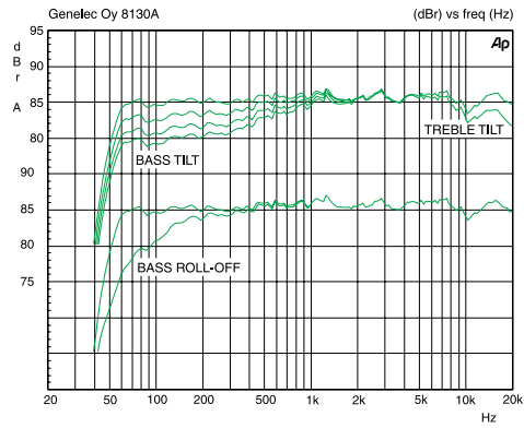
8130Aのフリーフィールド・レスポンスへのBASS TILT、TREBLE TILT、BASS ROLL-OFFの各コントロールの効果
