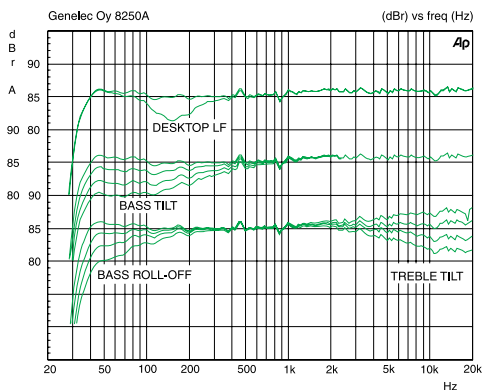
8250Aのフリーフィールド・レスポンスへのBASS TILT、TREBLE TILT、DESKTOP LOW FREQUENCY、BASS ROLL-OFFの各コントロールの効果
