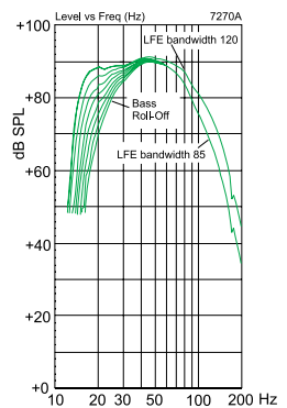
7260A/SE7261A (左)、7270A/7271A (右)のフリーフィールド・レスポンスへのBASS ROLL-OFFコントロールの効果
