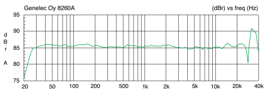
8260Aの軸上のフリーフィールド・レスポンス (40 kHz まで)
