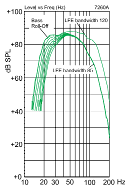
7260A/SE7261A (左)、7270A/7271A (右)のフリーフィールド・レスポンスへのBASS ROLL-OFFコントロールの効果
