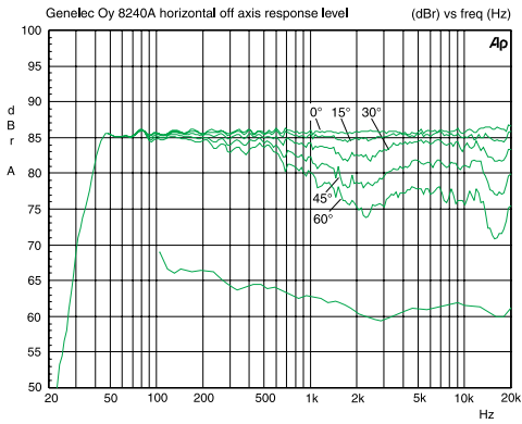
上側: 8240Aの水平指向性特性 (1 m 位置で計測)。下側: 同システムのパワー・レスポンス
