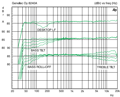
8240Aのフリーフィールド・レスポンスへのBASS TILT、TREBLE TILT、DESKTOP LOW FREQUENCY、BASS ROLL-OFFの各コントロールの効果
