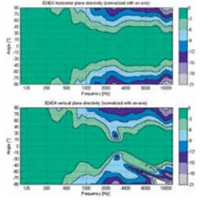
8240Aの水平指向性プロット (上)、垂直指向性プロット (下)
