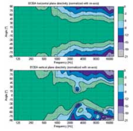
8130Aの水平指向性プロット(上)、垂直指向性プロット(下)
