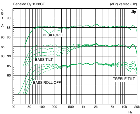
1238CFのフリーフィールド・レスポンスへのBASS TILT、TREBLE TILT、DESKTOP LOW FREQUENCY、BASS ROLL-OFFの各コントロールの効果
