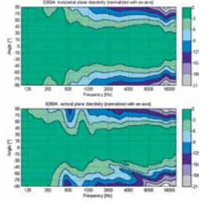
8260Aの水平指向性プロット (上)、垂直指向性プロット (下)
