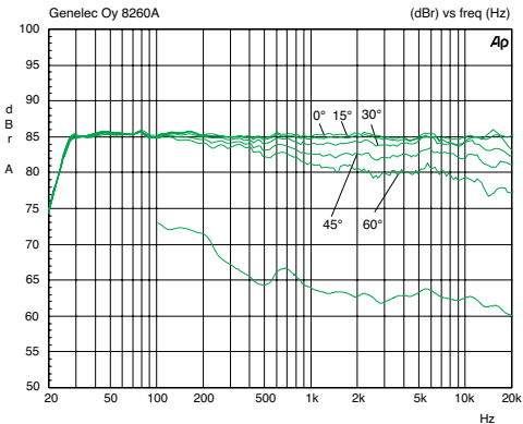
上側: 8260Aの水平指向性特性 (1 m 位置で計測)。下側: 同システムのパワー・レスポンス
