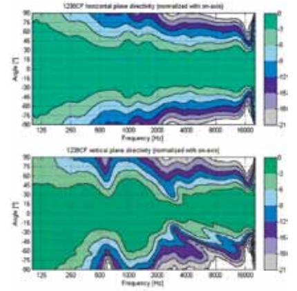
1238CFの水平指向性プロット(上)、垂直指向性プロット(下)
