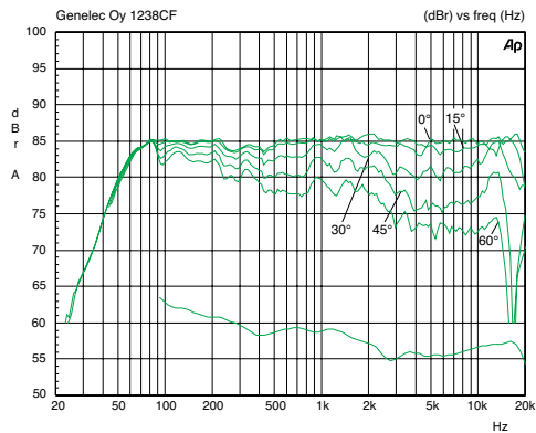
上側:1238CFの水平指向性特性(1m位置で計測)。下側:同システムのパワー・レスポンス
